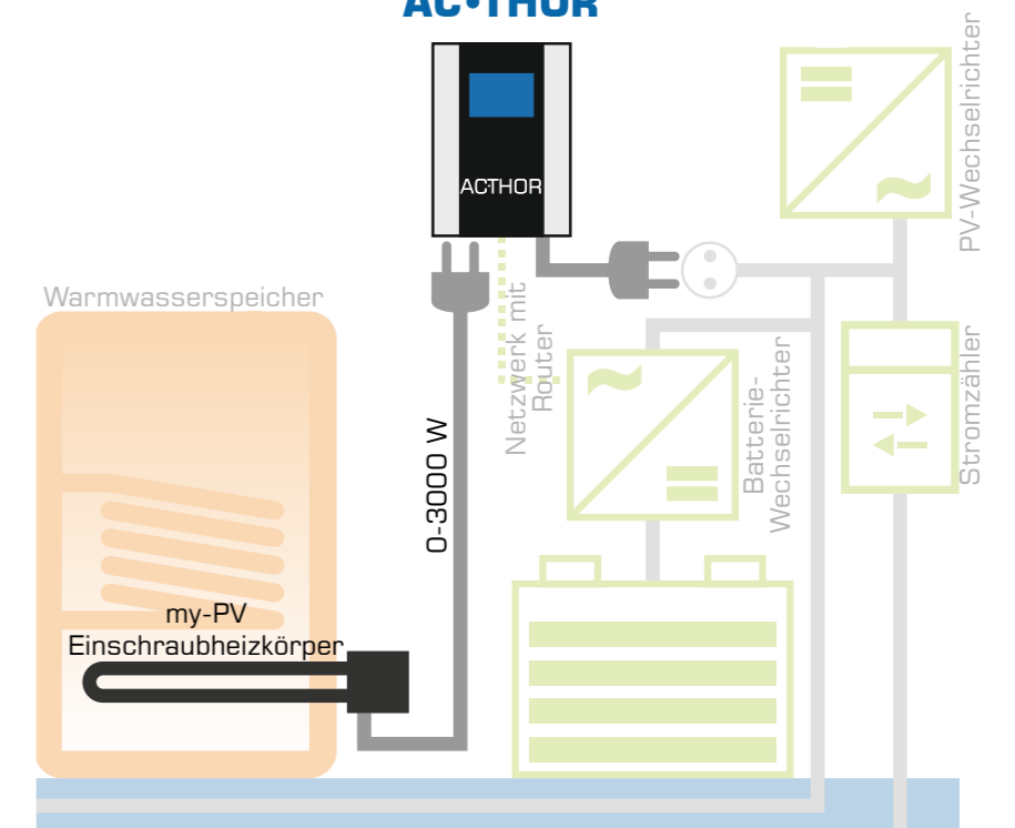
Mit Netzanbindung - mit Batteriespeicher
