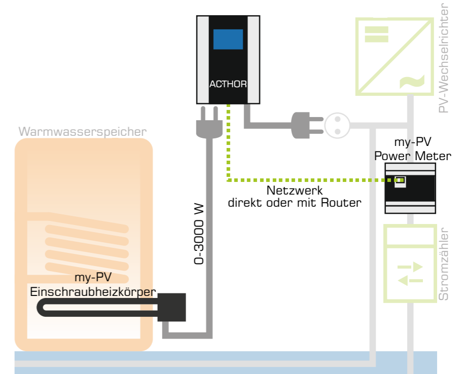
Mit Netzanbindung - ohne Batteriespeicher
