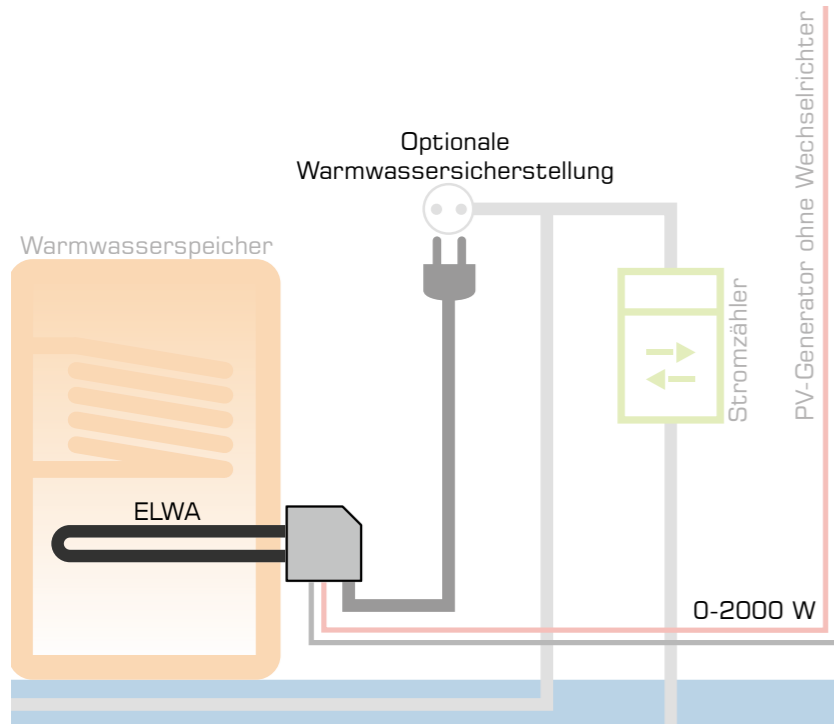
Ohne Netzanbindung - ohne Batteriespeicher
