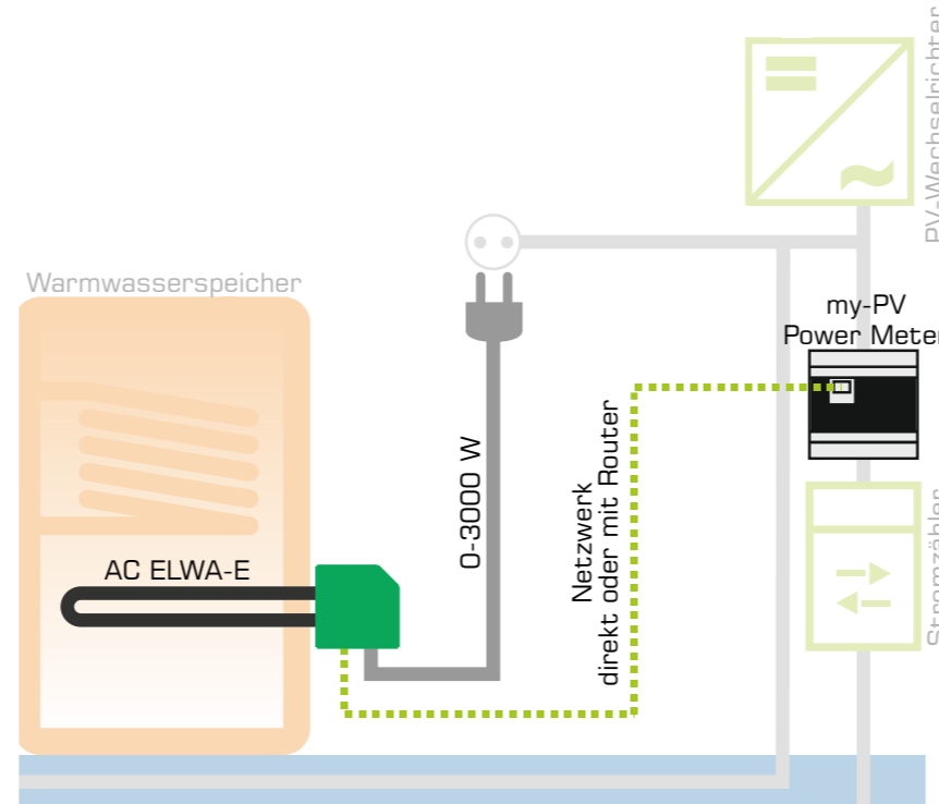
Mit Netzanbindung - ohne Batteriespeicher
