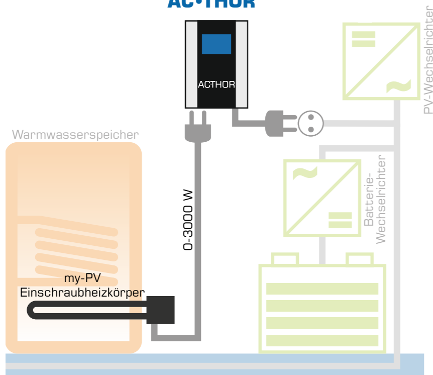
Ohne Netzanbindung - mit Batteriespeicher
