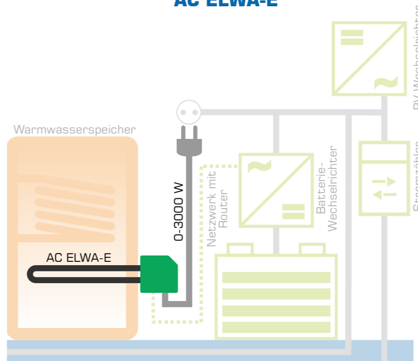
Mit Netzanbindung - mit Batteriespeicher
