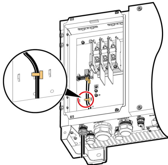
Abbildung 5-34 Binden der Kommunikationskabel
