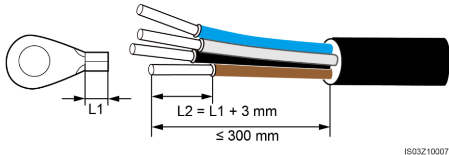
Abbildung 5-11 Vieradriges Kabel (ohne Erdungskabel, jedoch mit Neutralleiter)
