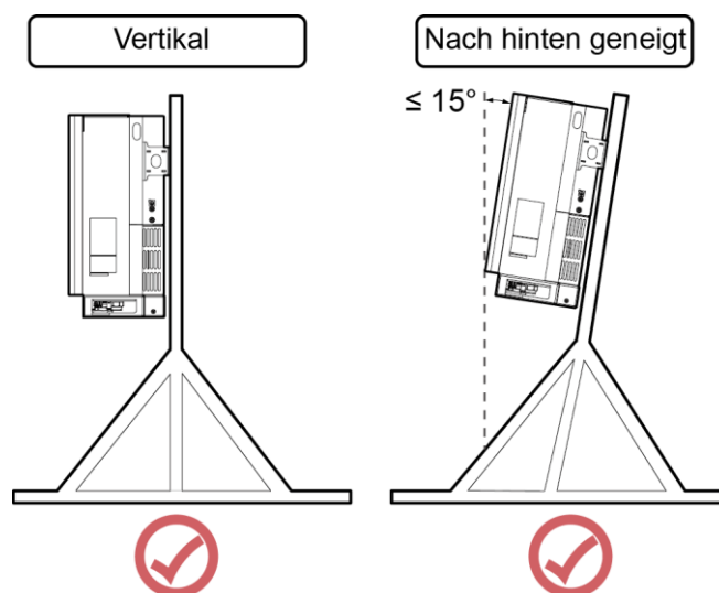
Abbildung 4-19 Richtige Montagewinkel
