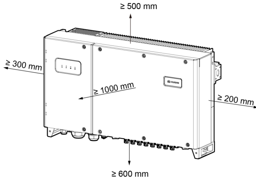
Abbildung 4-4 Montageabstände
