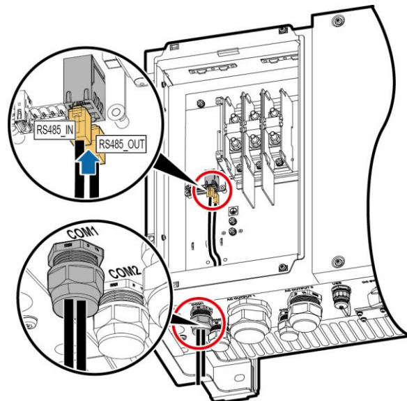
Abbildung 5-33 Anschließen der Kommunikationskabel
