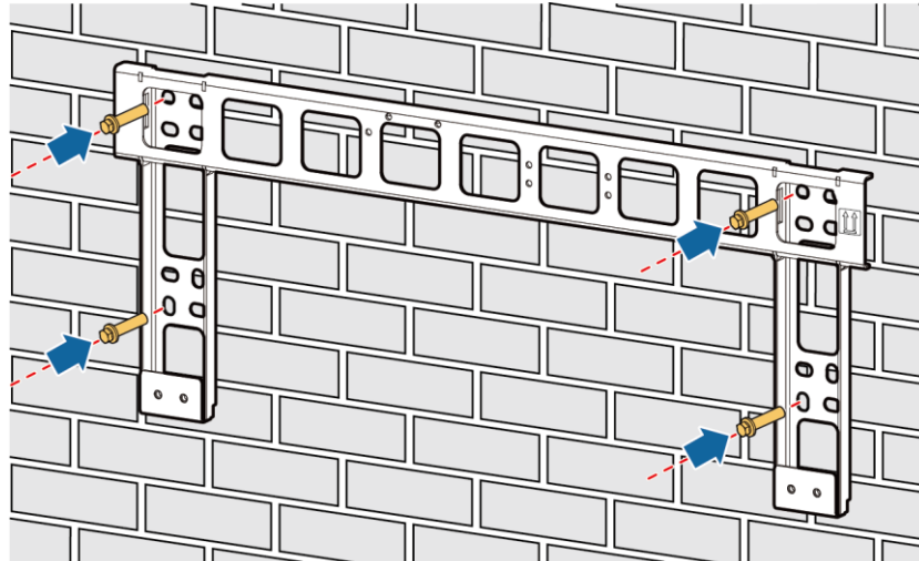
Abbildung 4-14 Befestigen einer Montagehalterung
