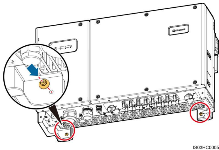
Abbildung 4-18 Anziehen von Torx-Sicherheitsschrauben
