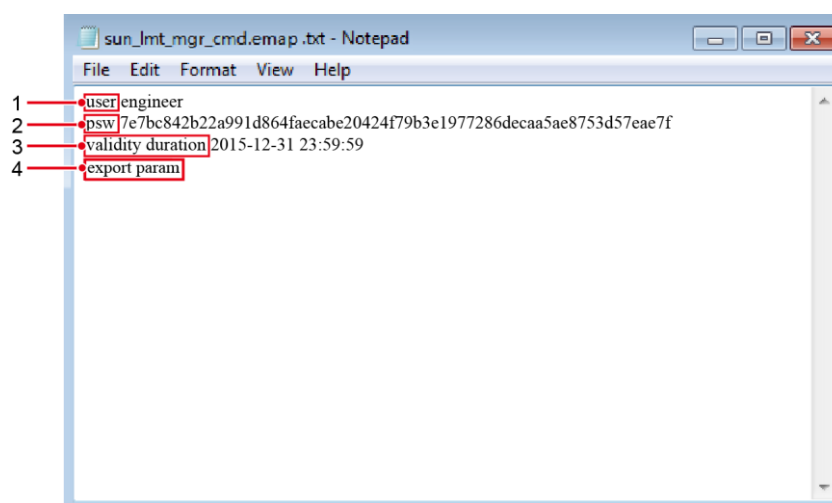
Abbildung 7-1 Boot-Skriptdatei
