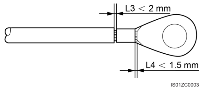
Abbildung 5-4 Crimpen eines Kabels
