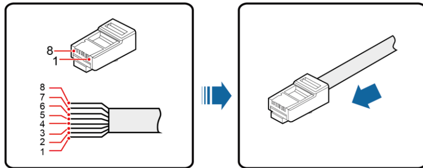
Abbildung 5-32 Anschließen der Adern an einen RJ45-Steckverbinder
