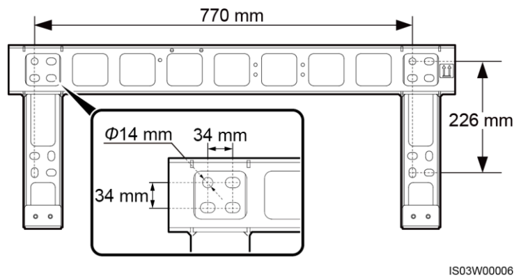
Abbildung 4-22 Abmessungen der Montagehalterung
