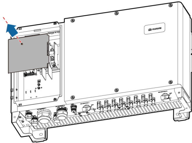
Abbildung 5-7 Entfernen der Abdeckung des AC-Klemmenblocks
